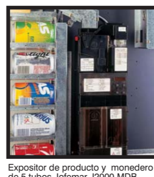
Expositor de producto y monedero de 5 tubos Jofemar J2000 MDB. Product display and Jofemar J2000 MDB, 5 tubes coin changer.
